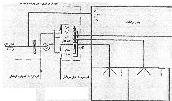
سیستم CAV چند زونه با سه پلنوم
