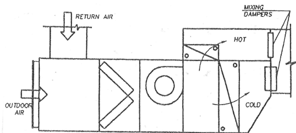
هواساز حجم ثابت چند زونه CAV-MZ
