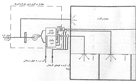
سیستم CAV چند زونه با کویل بازگرمایش
