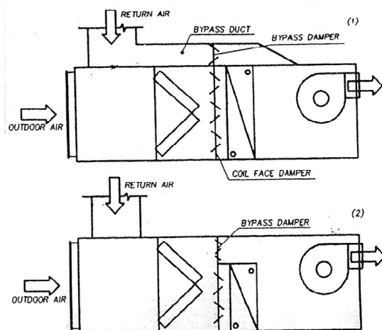
شکل (۱-۲) کنترل دمپر رخ و کنارگذر
